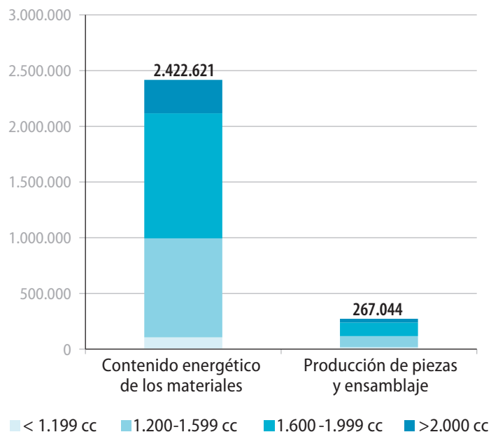
Figura 44. Consumo energético en la fabricación (producción de materiales y ensamblado) de turismos en España en tep (2012)
